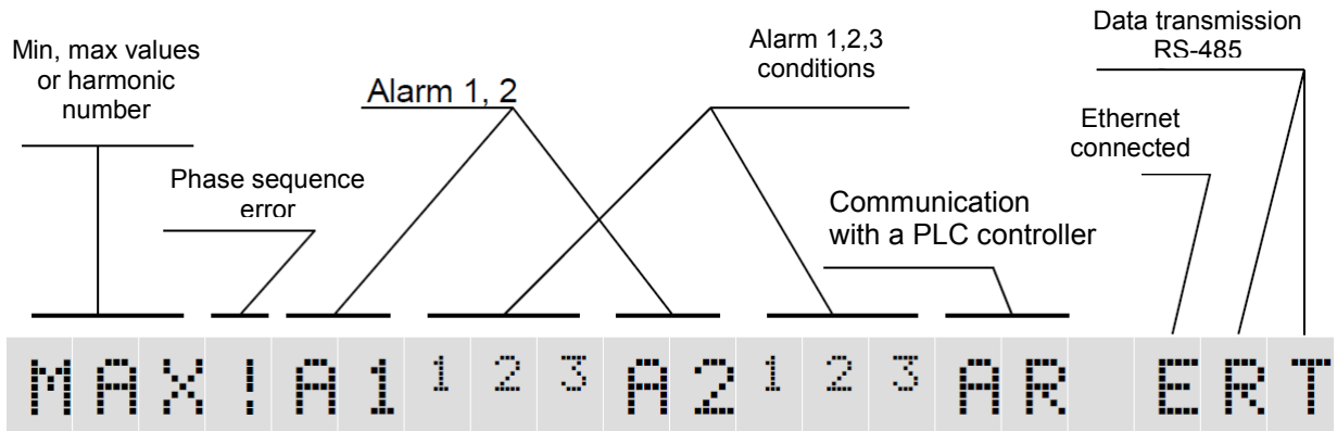
Fig.10. Information bar
